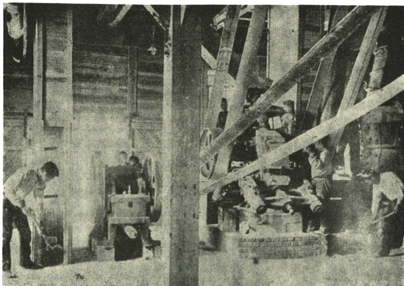
北陸人造肥料株式会社の製造場
